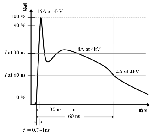
図1 ESD 試験器の電流波形 (IEC61000-4-2)
