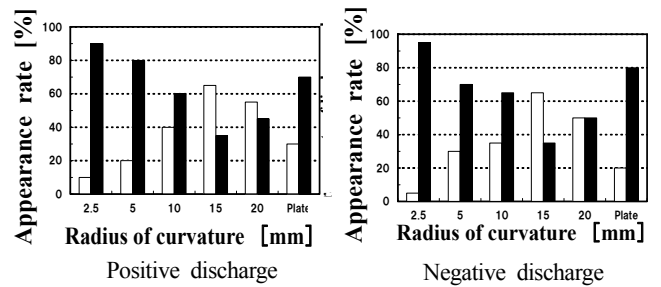
(b) 2種類の放電路の出現率と接地電極の曲率半径 (人体電位: \pm 4\text{kV} )
