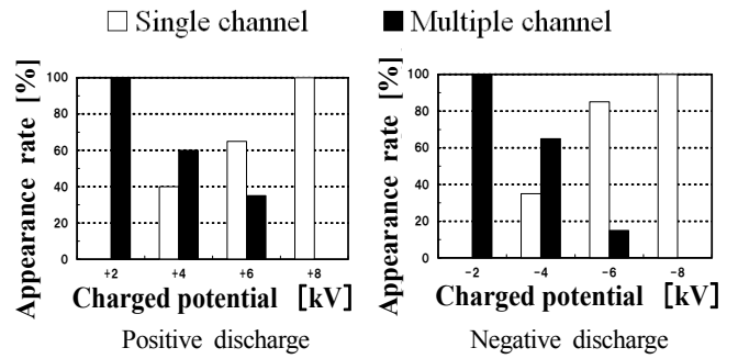
(a) 2種類の放電路の出現率と人体電位 (接地電極の曲率半径: 10 mm)
